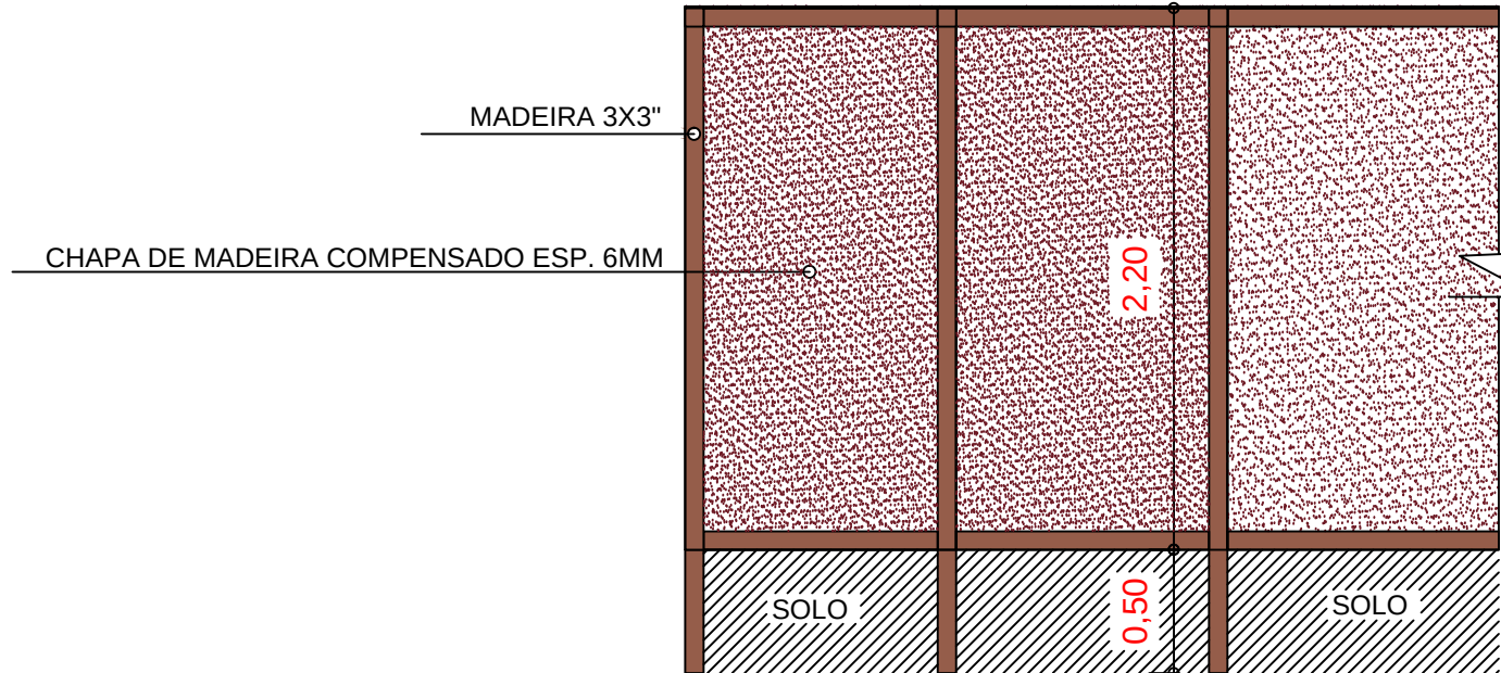
DETALHE TAPUMES
