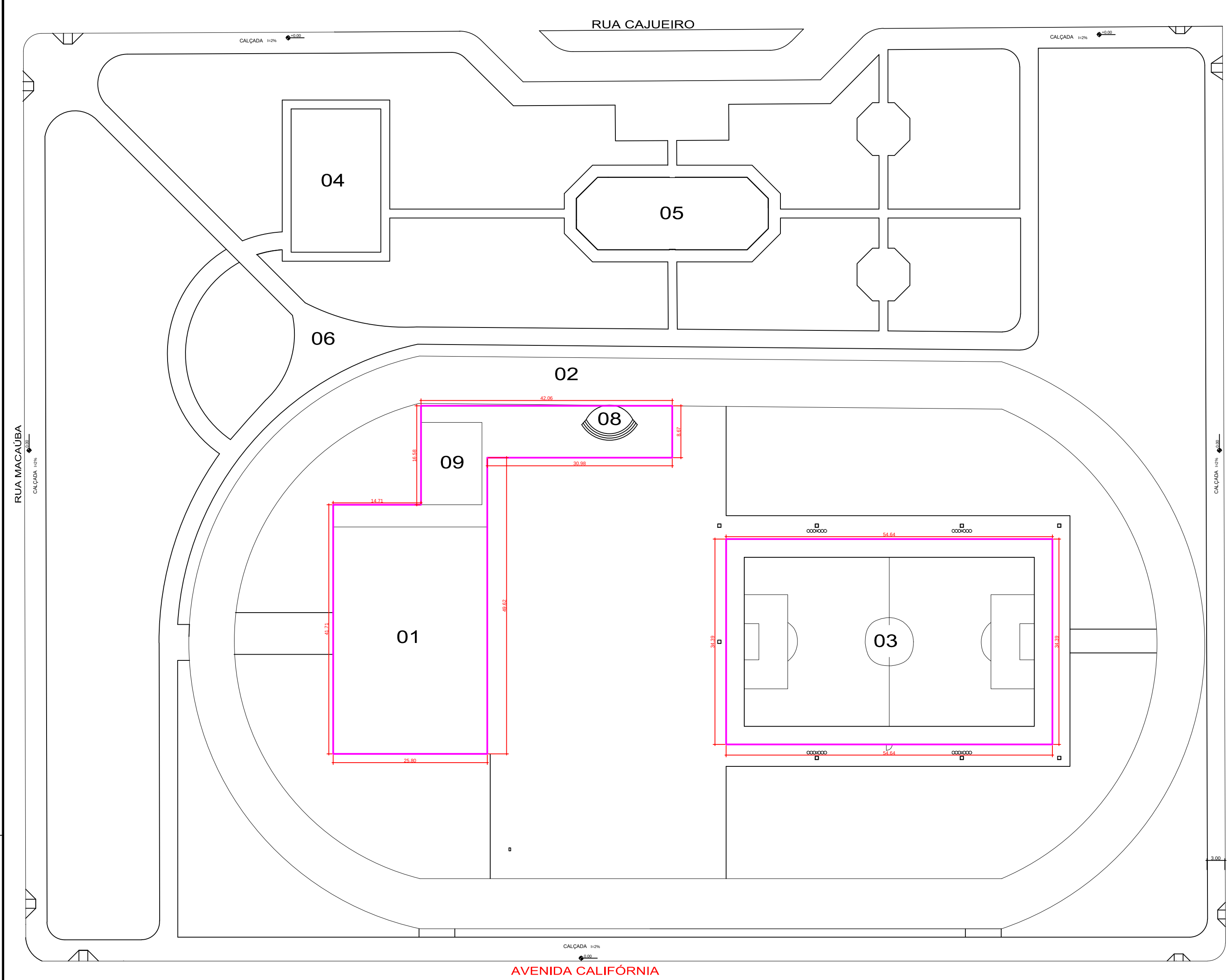
LOCAÇÃO TAPUMES
